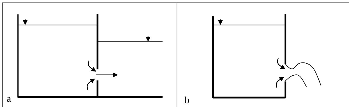
Fig. (IV.1) : (a) : orifice noyé, (b): orifice non noyé.
