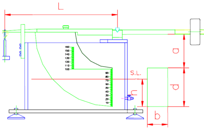
Figure 1 : Dimensions de l'appareil.
