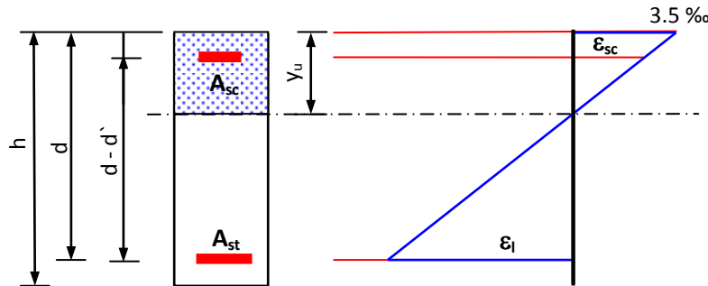
Fig. 5.6 : Diagramme de déformation
