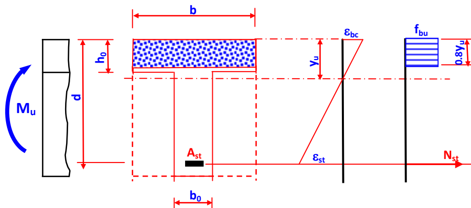
Fig. 5.8: Principe de calcul à l'ELU d'une section en T, avec : M_t \geq M_u
