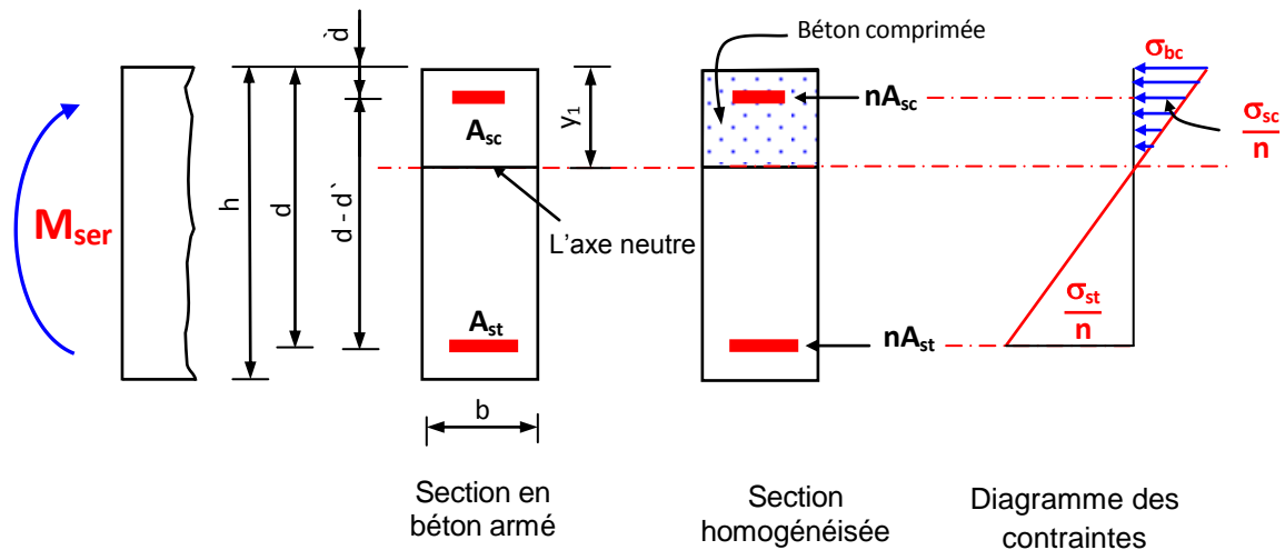
Fig. 5.12 : Section rectangulaire avec armatures comprimées.
