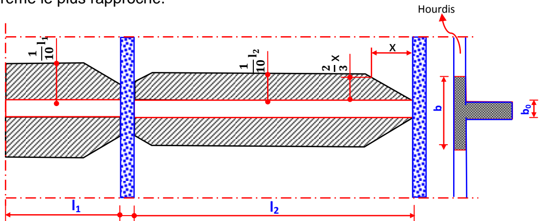
Fig. 5.7 : Largeur de la table de compression
