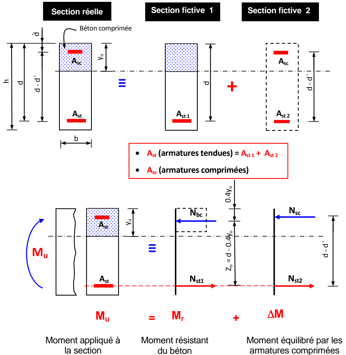
Fig. 5.5 : Principe de calcul à l'ELU d'une section rectangulaire avec aciers comprimés
