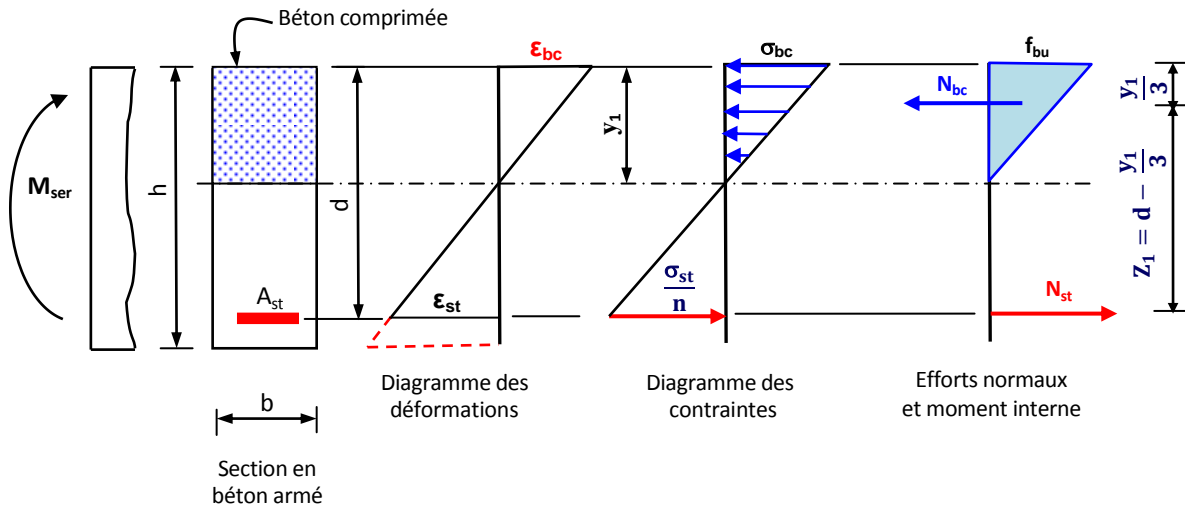
Fig. 5.11 : Principe de calcul à l'ELU d'une section en T avec aciers comprimés
