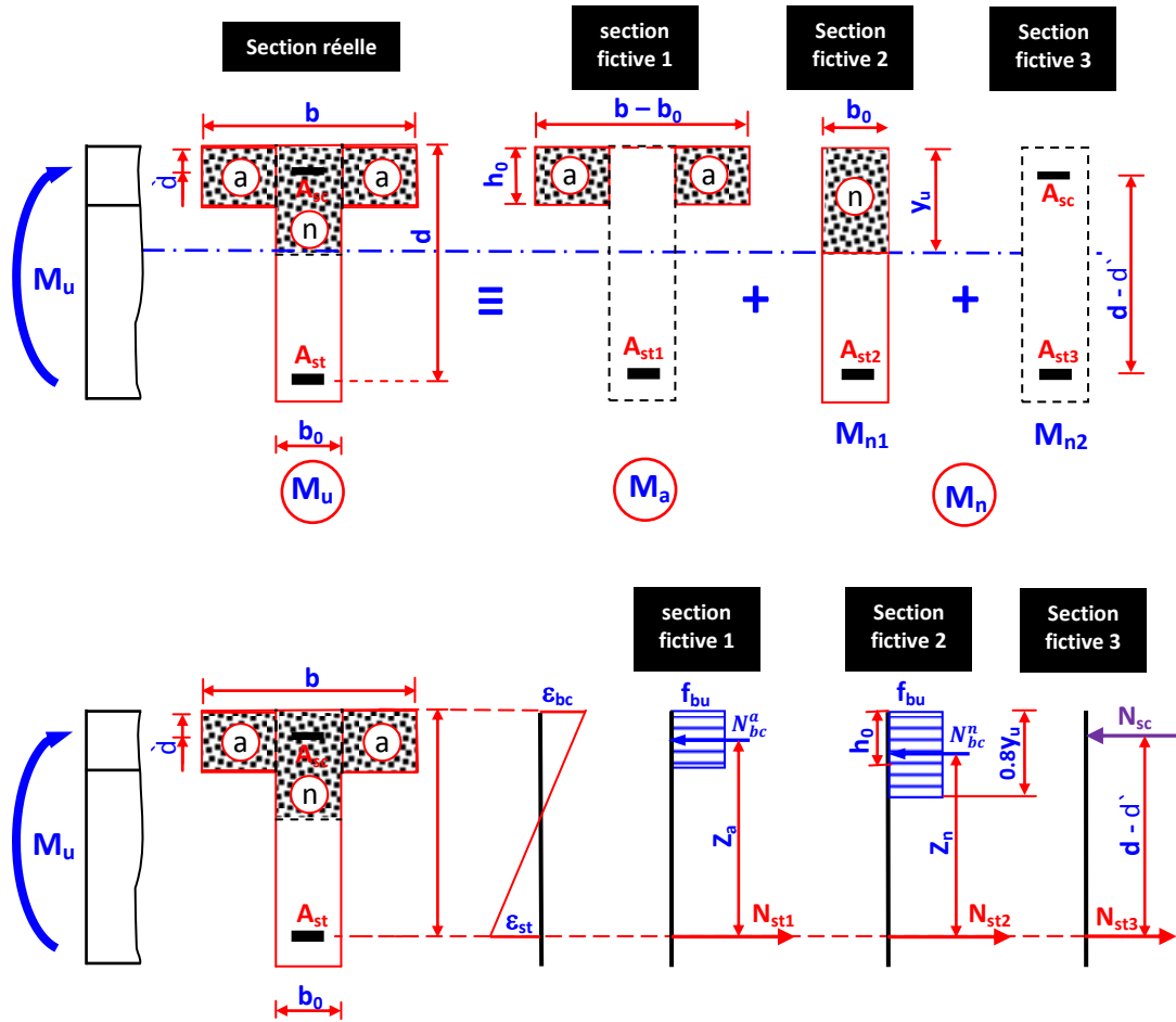
Fig. 5.10 : Principe de calcul à l'ELU d'une section en T avec aciers comprimés
