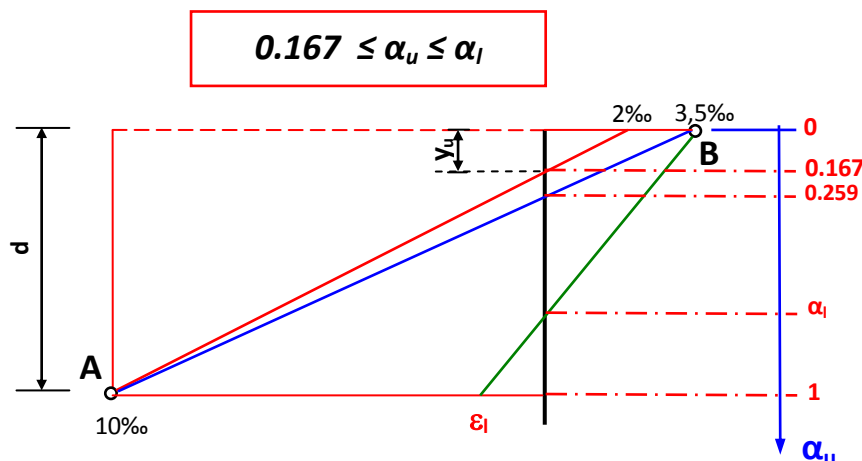
Fig. 5.3: Positions particulières de l'axe neutre
