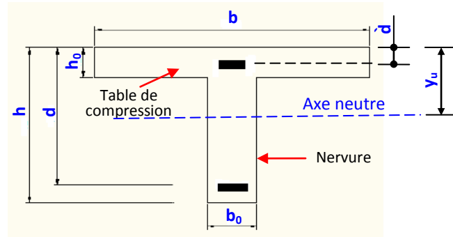
Fig. 5.6 : Élément en béton armé de section en forme d'un té
