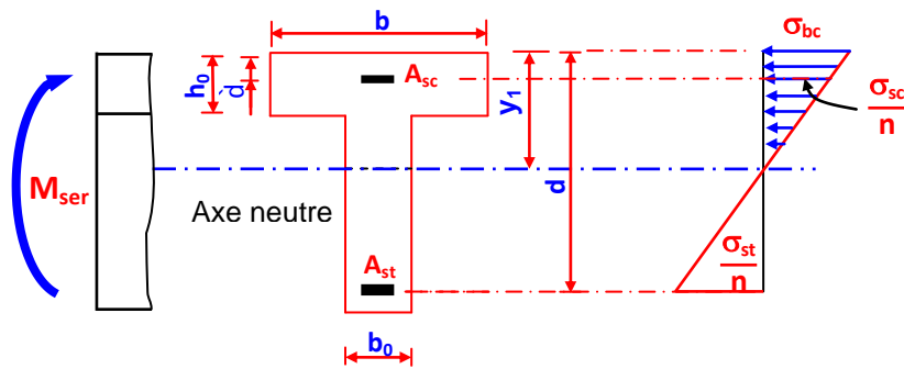
Fig. 5.13 : Section en T avec armatures comprimées.
