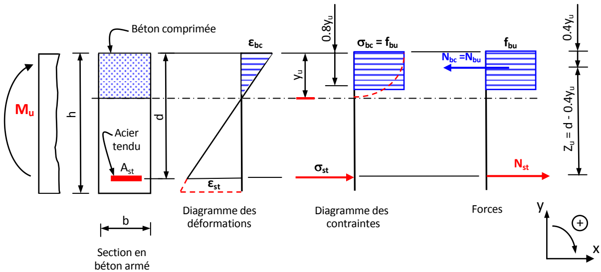
Fig. 5.4 : Diagrammes contrainte-déformation parabolique-rectangulaire et rectangulaire simplifié dans la section de béton comprimé
