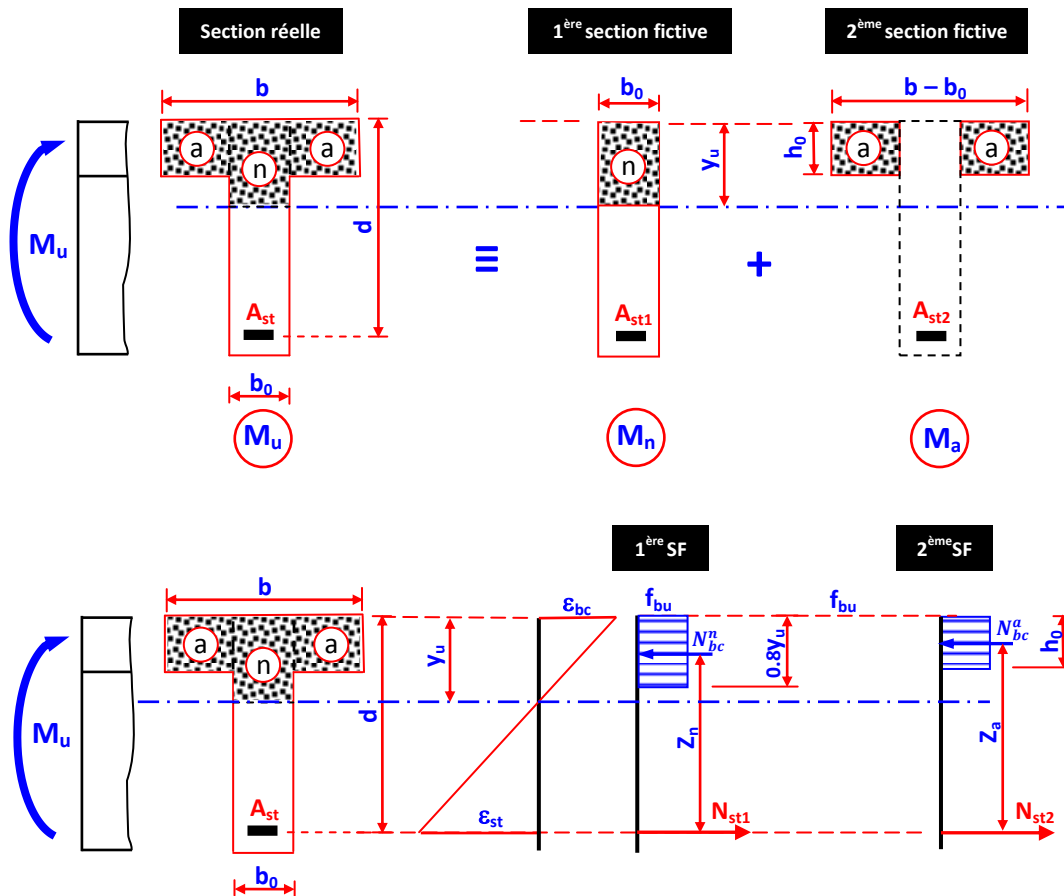
Fig. 5.9: Principe de calcul à l'ELU d'une section en T, avec : M_t < M_u
