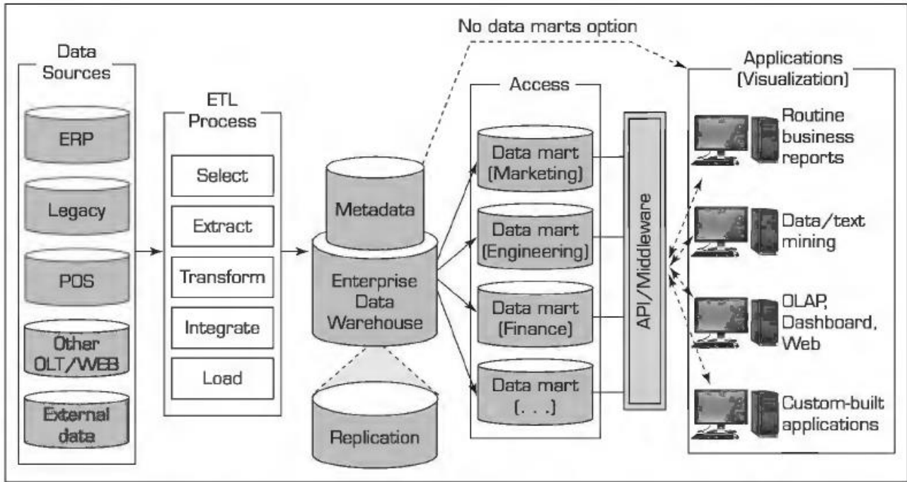
الشكل رقم (01): إطار عمل مستودع البيانات
