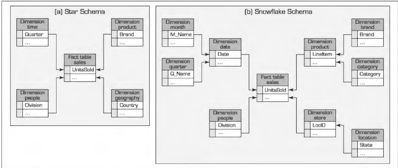
(a) The Star Schema, (b) the Snowflake Schema: (02) الشكل رقم
