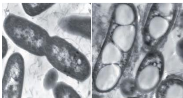
Fig. 2: a) Cellules bactériennes normales. b) Production de polyester (PHA) au sein de cellules bactériennes.
