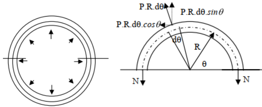
Figure 5.3. Tirant circulaire
